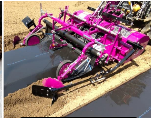
溝浚板ASSY5型 食い込み性が良く、作業中に 浮き上がりにくい改良型です。
